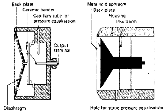
شکل شماره ۲- نمایشی از ساختار میکروفن کریستالی
