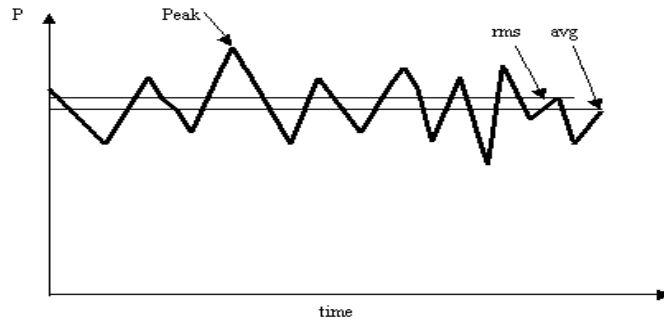
شکل شماره ۵- مقایر حداکثر، مؤثر و میانگین فشارها در يك دوره زمانی
