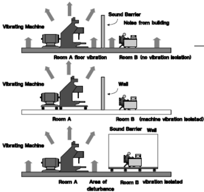
شکل شماره ۳- نمایی از ایزولاسیون ارتعاش دستگاه به اشکال مختلف
